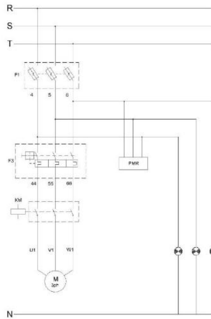
شکل ۱۸) نمای شماتیک مدار قدرت WA 90-120
