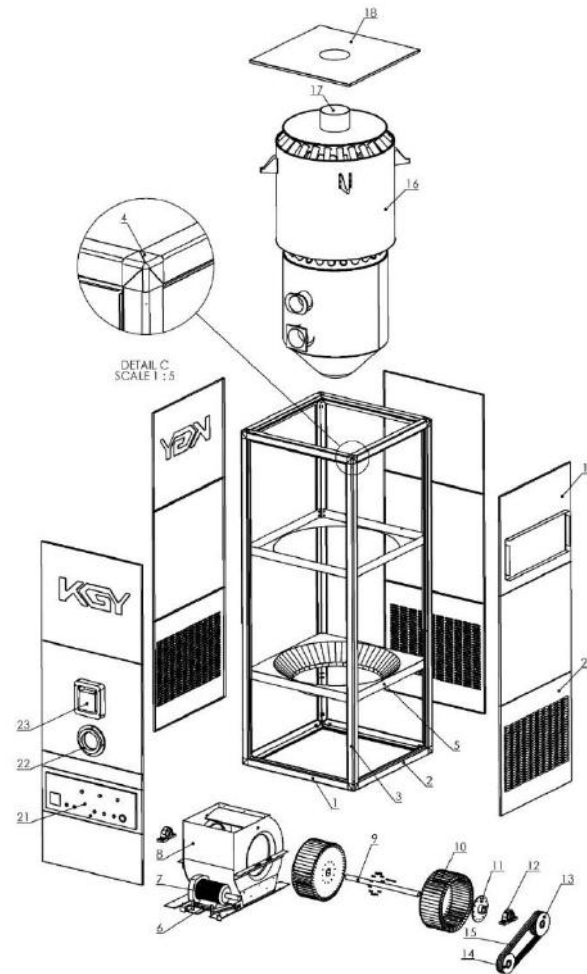
شکل ۱۰ نقشه انفجاری هیتر
