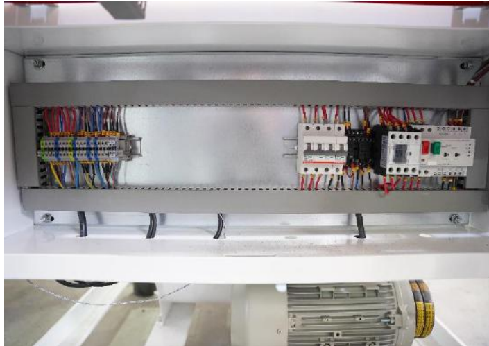
شکل (۱۱) تابلو برق دستگاه
