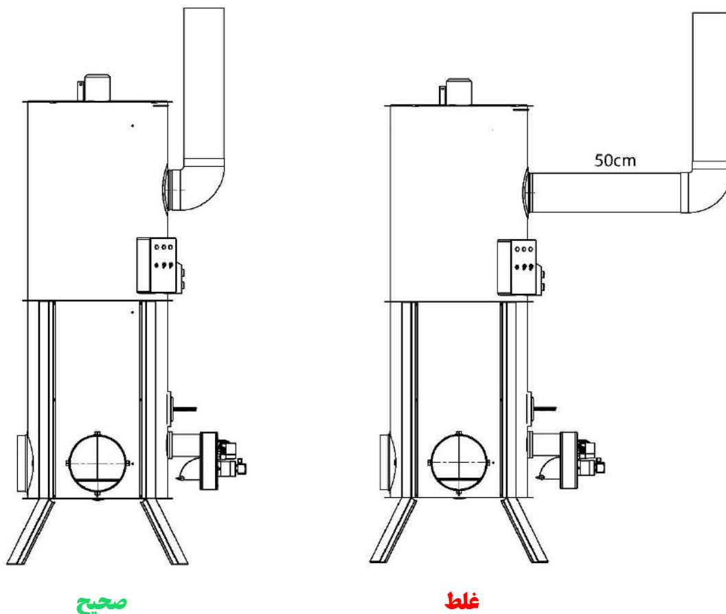
شکل ۷) نصب دودکش
